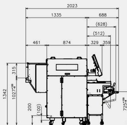
Vista lateral
