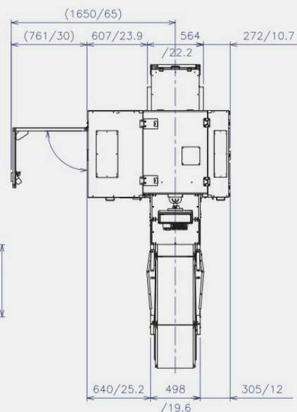
Vista superior
