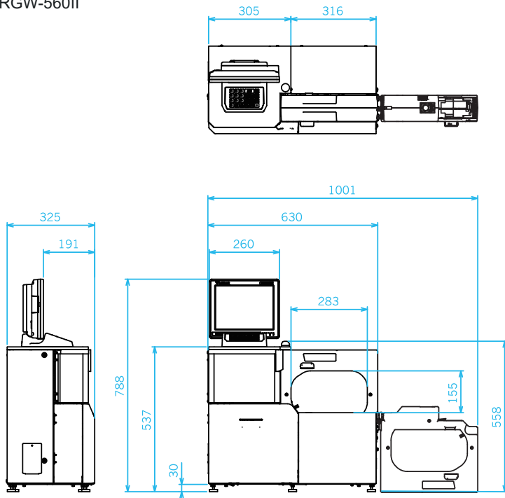
Configuración con consola RGW-560II
