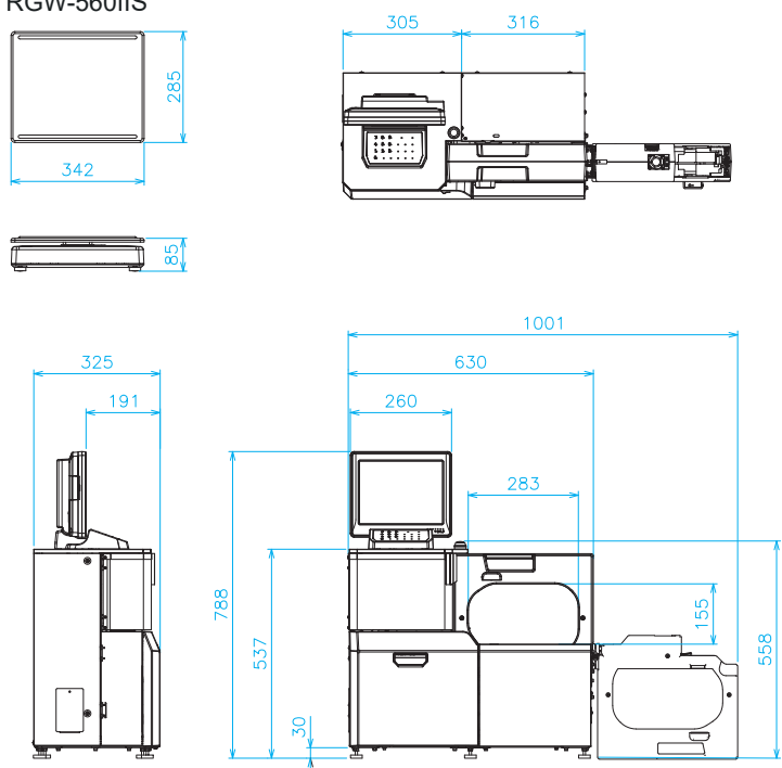
Configuración con consola y balanza RGW-560IIS
